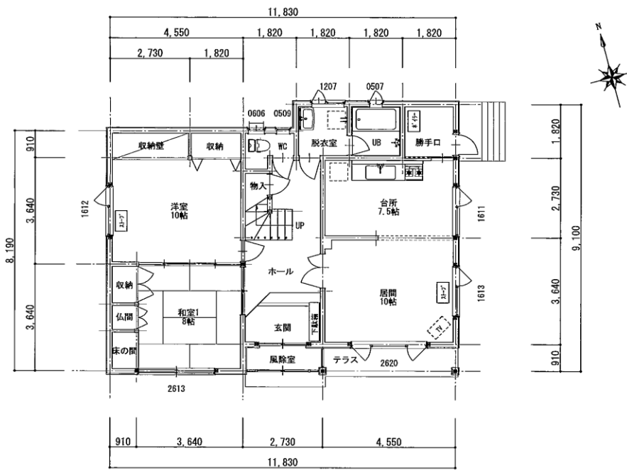
1階平面図 S=1/100 (参考図)
