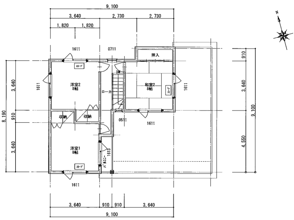
2階平面図 S=1/100 (参考図)
